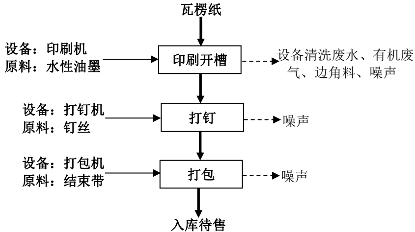
图 2-5 本项目普通纸箱生产工艺流程及产污环节图
