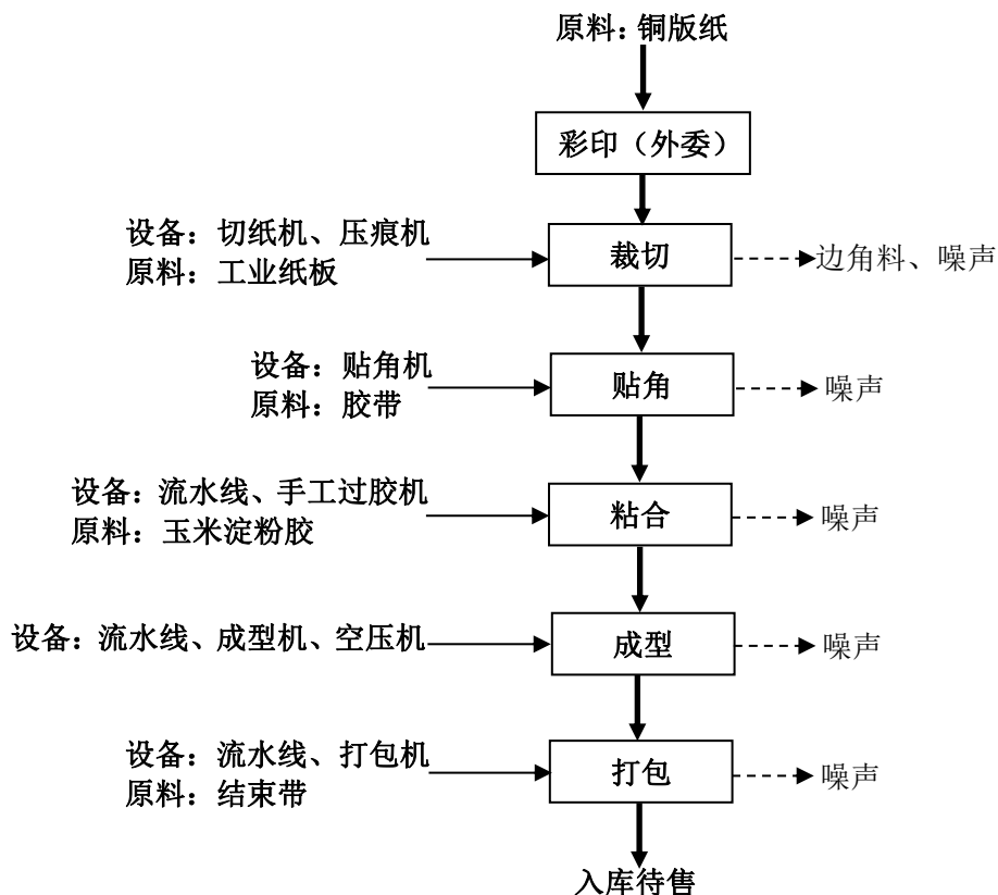
图 2-4 本项目鞋盒产工艺流程及产污环节图
