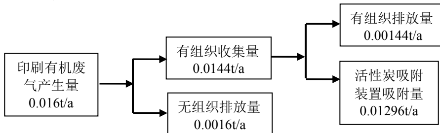
图 4-1 本项目 VOCs 平衡图
