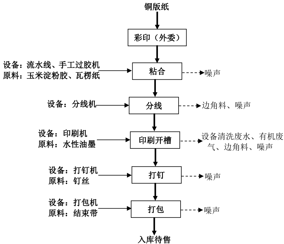
图 2-6 本项目彩色纸箱生产工艺流程及产污环节图
